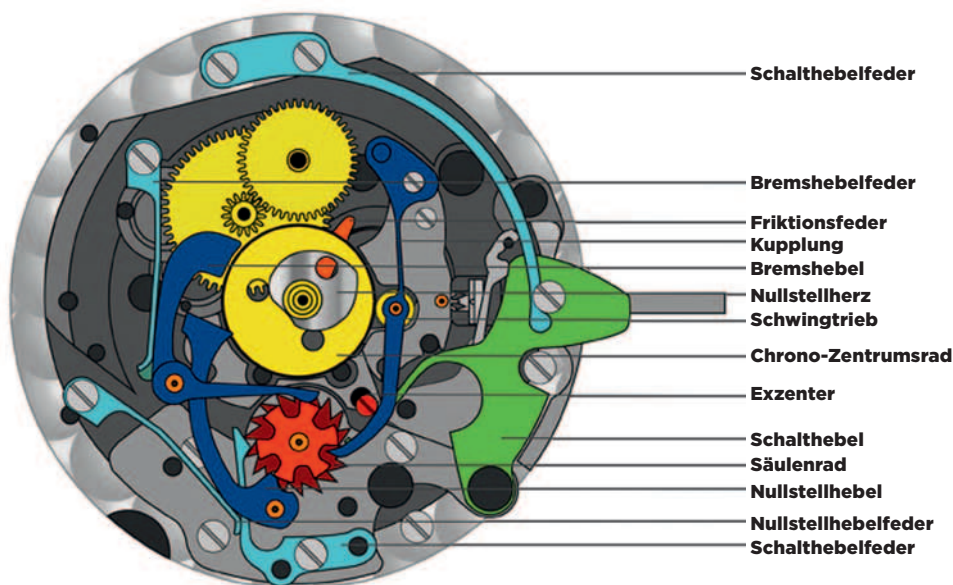
Funktionszeichnung: Blick auf ein Chronographenwerk mit Schaltradsteuerung.
